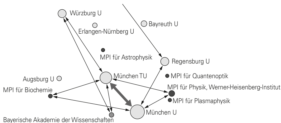
Abbildung 2: Physik
